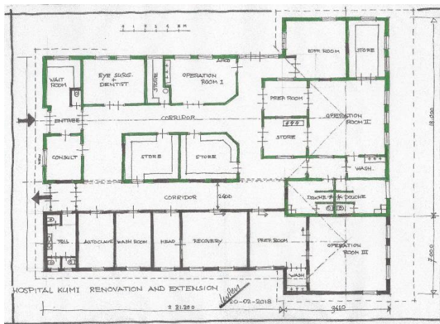
Renovatie en uitbreidingsplan Kumi Hospitaal
